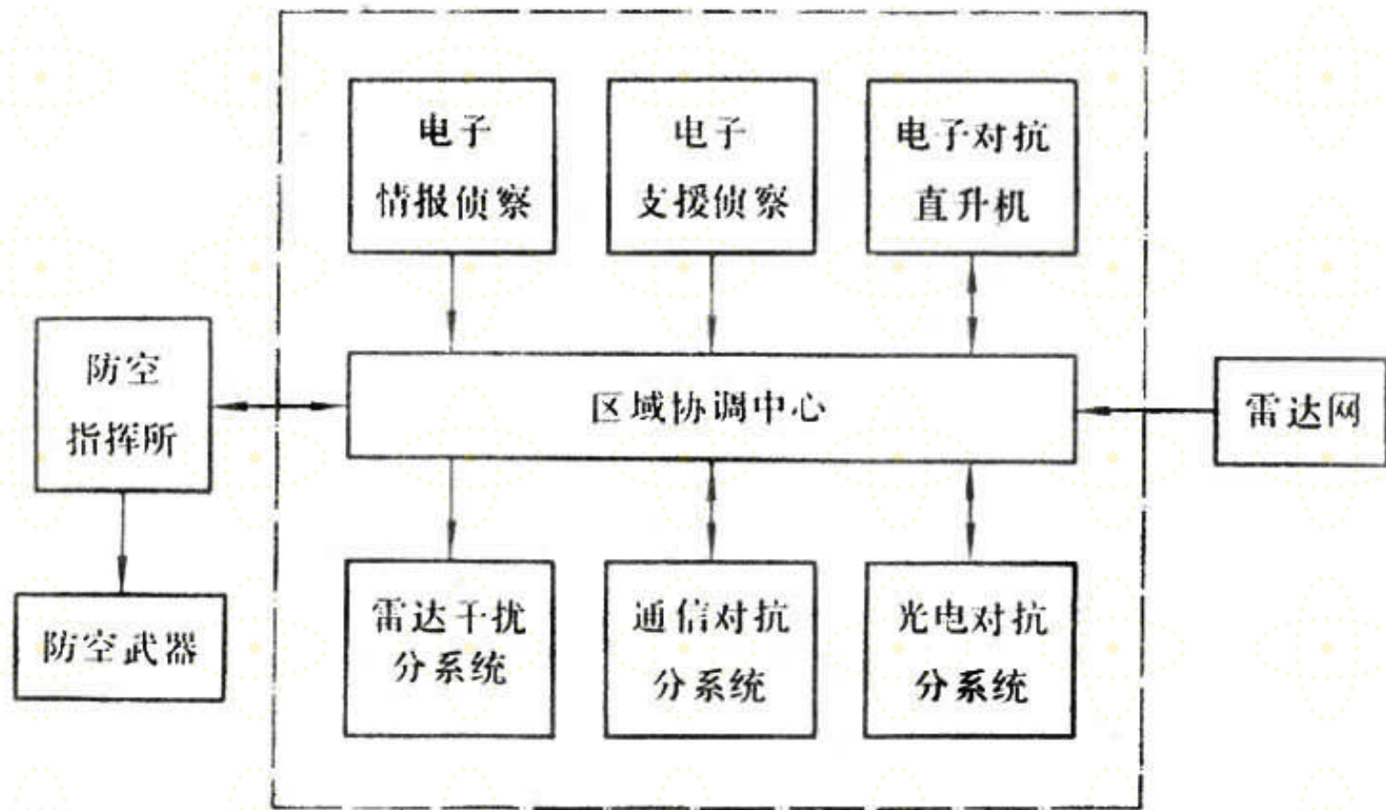
图 1 防空电子对抗系统组成框图
